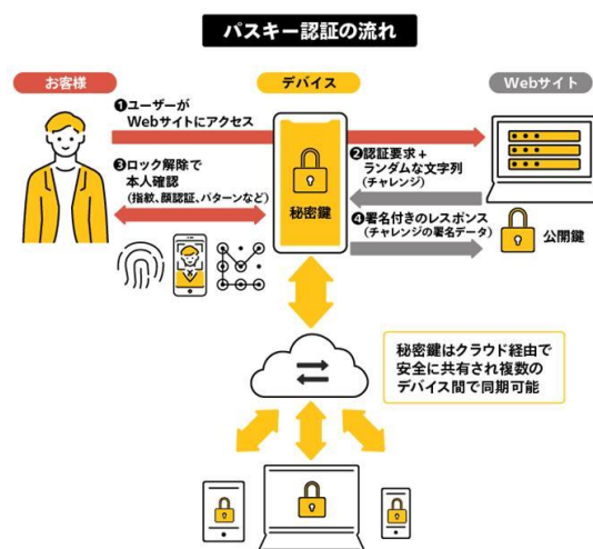
図 1：パスキー認証の流れ（※1）
